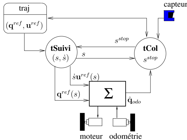
FIG. 5.5 – Architecture de contrôle de suivi de trajectoire et de l'évitement d'obstacles.
