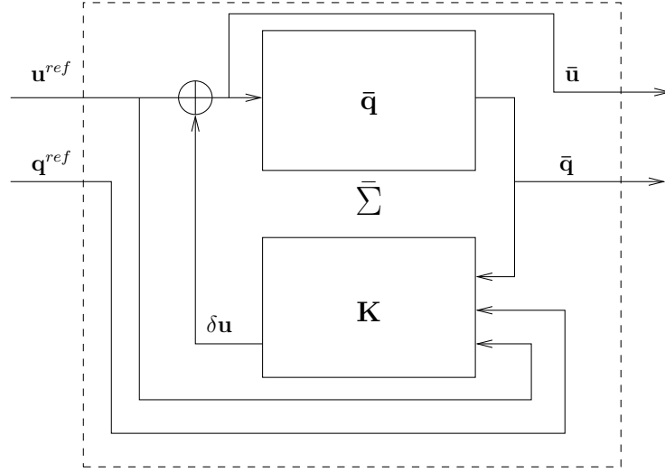
FIG. 5.10 – Module de simulation ( \bar{\Sigma} ) du système ( \Sigma ). L'entrée est une trajectoire de référence ( \mathbf{q}^{ref}, \mathbf{u}^{ref} ) non nécessairement admissible. La sortie est une trajectoire admissible ( \bar{\mathbf{q}}, \bar{\mathbf{u}} ).
