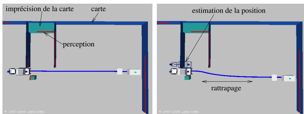
FIG. 6.5 – Suivi de trajectoire sans collision. Le rattrapage de la trajectoire n'est pas réalisé dès la discontinuité de la localisation, mais est reporté en «aval» sur la trajectoire.
